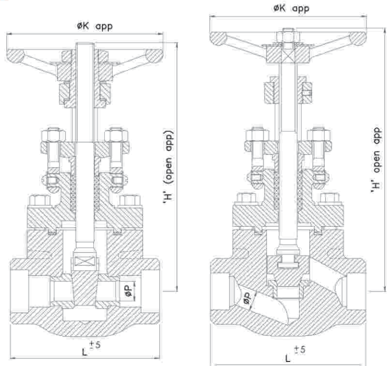
CLASS 800 FIG SV F1080
