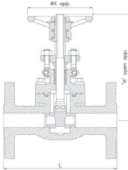
FIG SV1015WF - 1030WF - 1060WF
