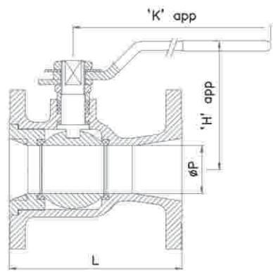
CLASS 150 FIG SV50151R
