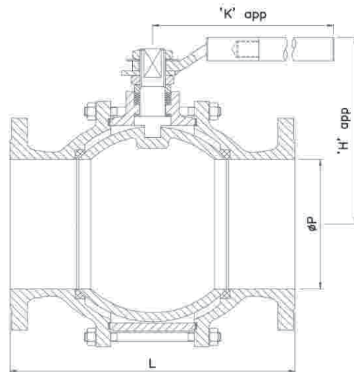
CLASS 150/300 3PIECE FIG SV50153F
