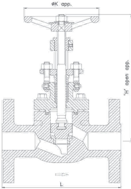
FIG SV2015WF - 2030WF - 2060WF
